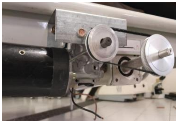
Gambar 5. Sistem penggerak motor menggunakan belt
